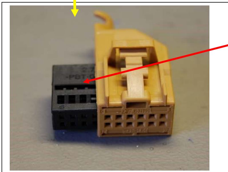
Kontaktträger
