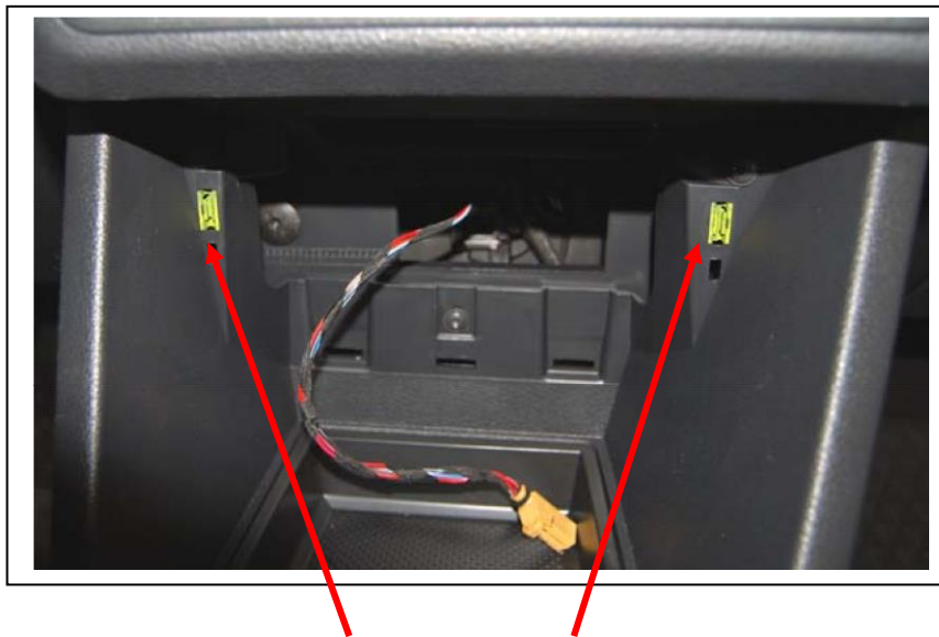
Halteklammern für Tasterrahmen (Rahmen ist auf dem Foto bereits entfernt)
